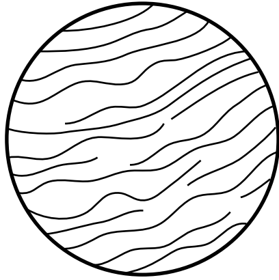
Venus
