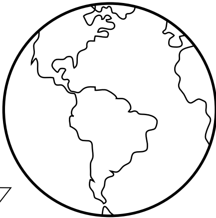
Terre
