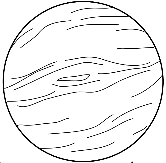
Jupiter
